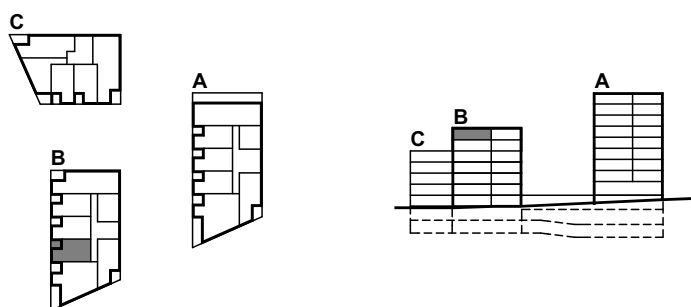
BLOK B, 7. PODLAŽÍ
